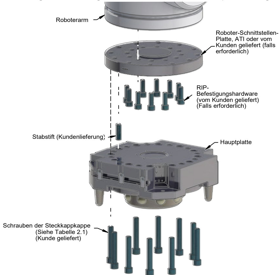
Abbildung 3.1—Werkzeugwechsler zur Roboterinstallation (QC-310 dargestellt)
