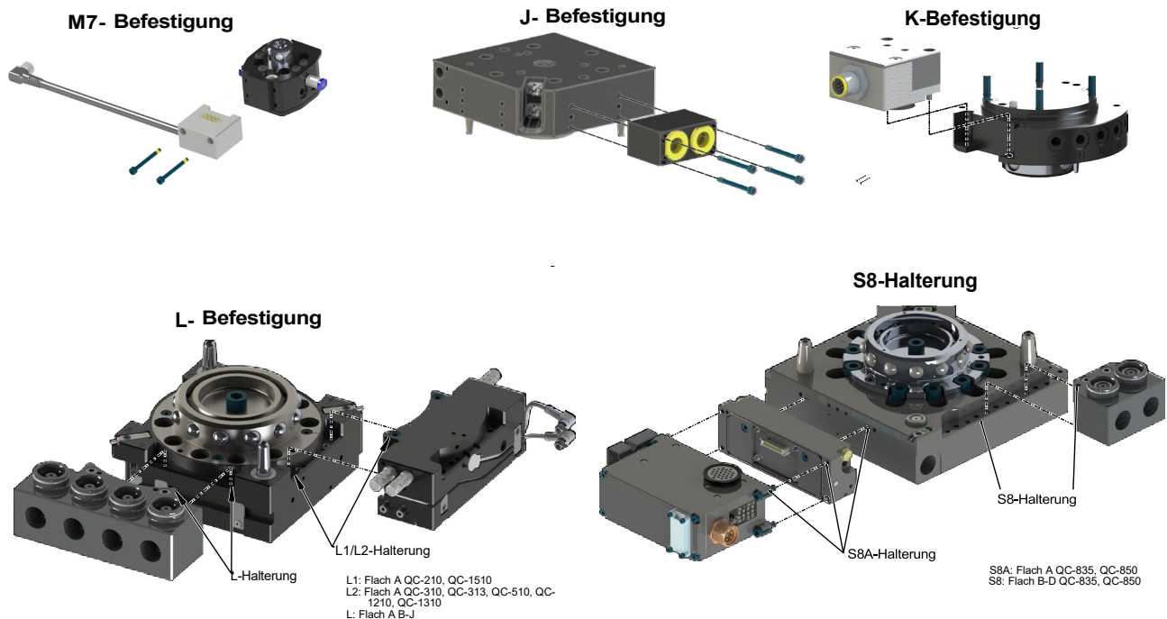
Abbildung 3.3 – Befestigungsarten für ATI-Module
